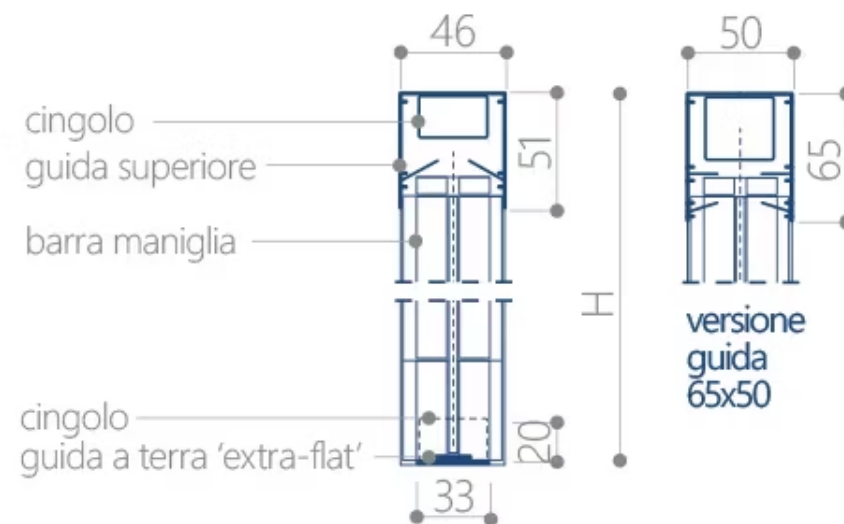
sezione verticale
